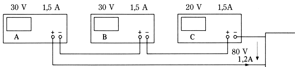
Fig. 9. Serieforbindelse af tre SN17-enheder
